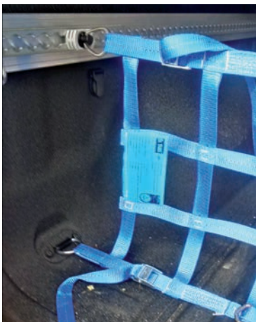
Détail des fixations latérales
